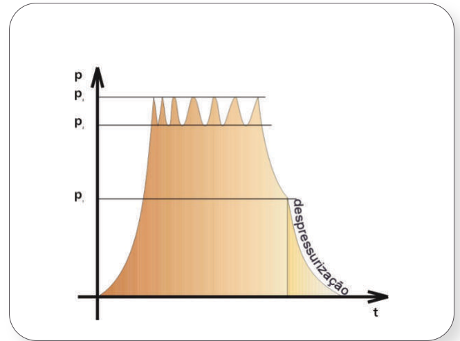
Pressões durante transporte por fase densa Dense phase conveying pressure behavior Presiones durante transporte por fase densa
