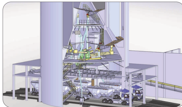
Silo de cone invertido / Inverted Cone Silo / Silo de cono invertido
