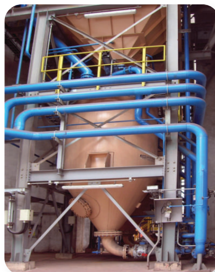
Transporte pneumático em fase densa Pneumatic conveying dense phase Transporte neumático en fase densa
