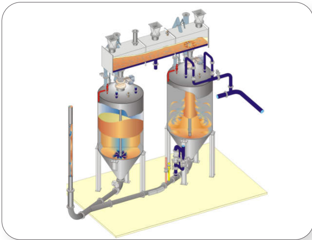
Pressões durante transporte por fase densa Dense phase conveying pressure behavior Presiones durante transporte por fase densa
