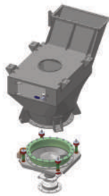
Moega fechada e descarregador vibratório Closed Hopper and vibratory discharger Tolva encerrada y descargador vibratorio
